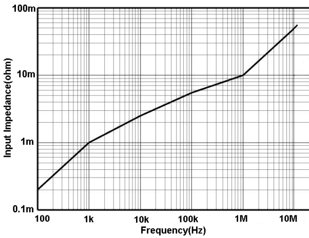
图 6 SCP5150 输入阻抗 VS 频率曲线
