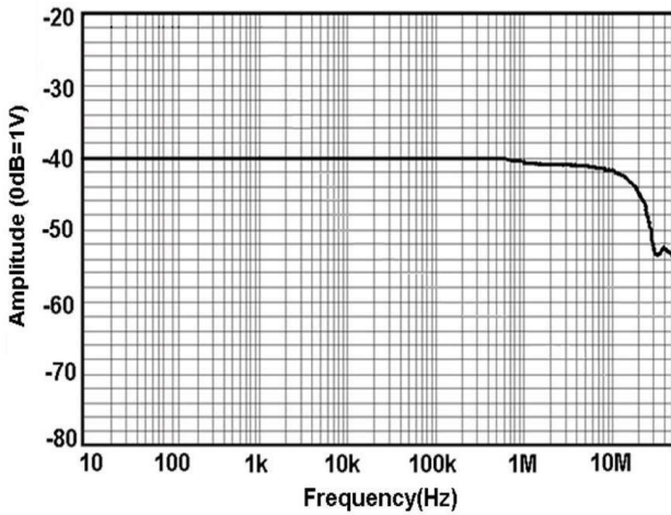
图 4 SCP5150 幅频曲线
