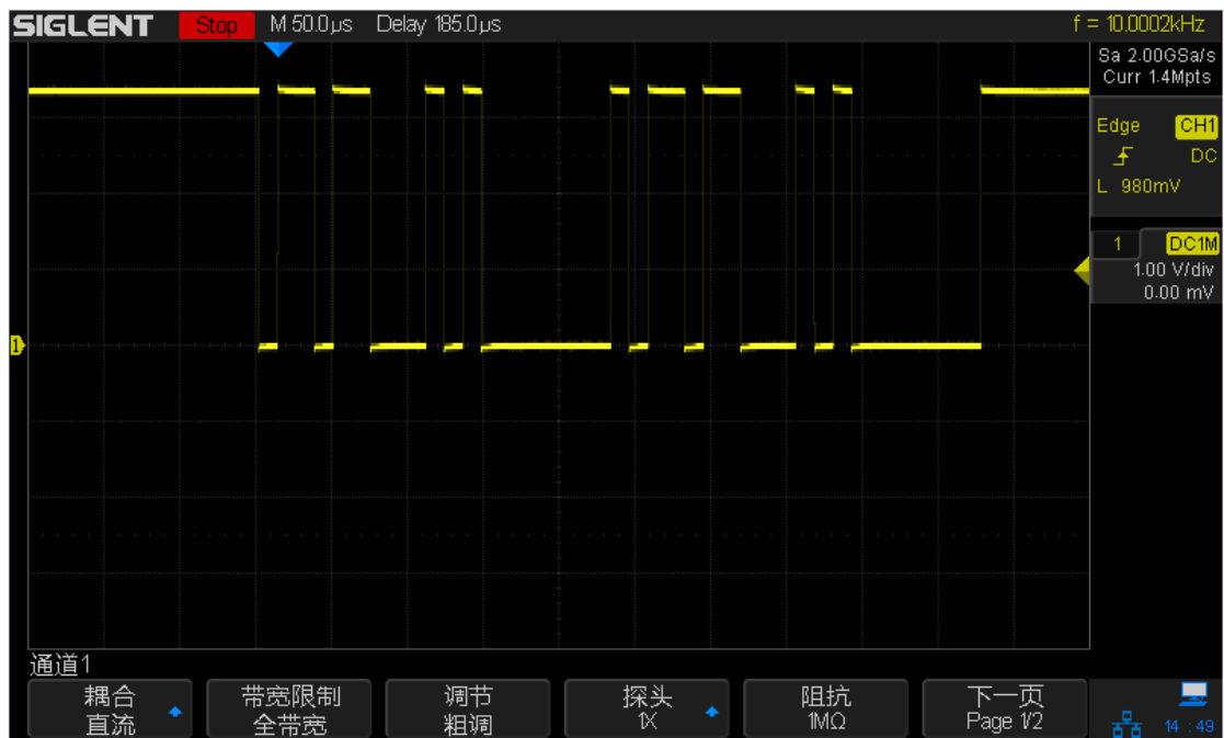
图 2.发送波形后波形发生器输出已编辑的任意波形
