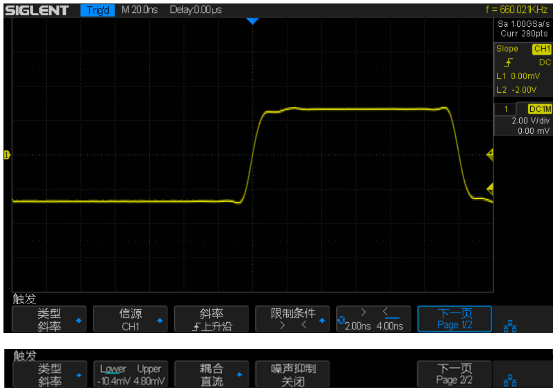
图 35 斜率触发
