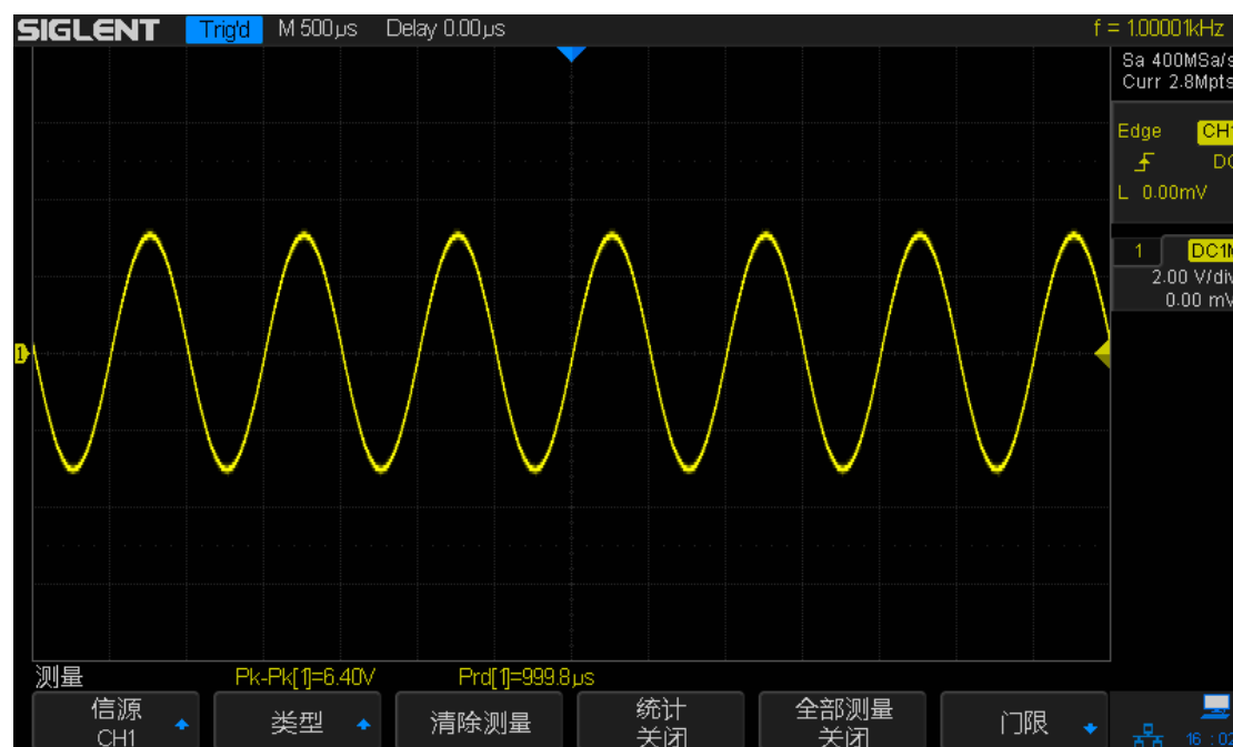
图 89 一键测量
