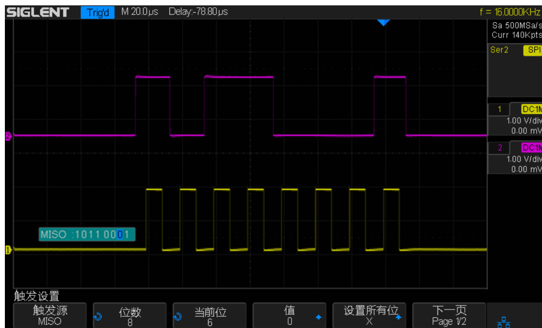
图 57 SPI 触发图
