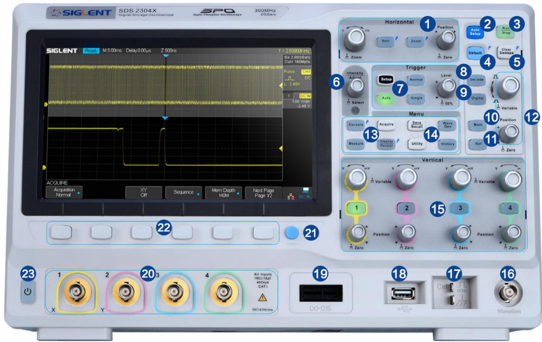
图 6 前面板总览
