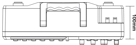
图 2 俯视图
